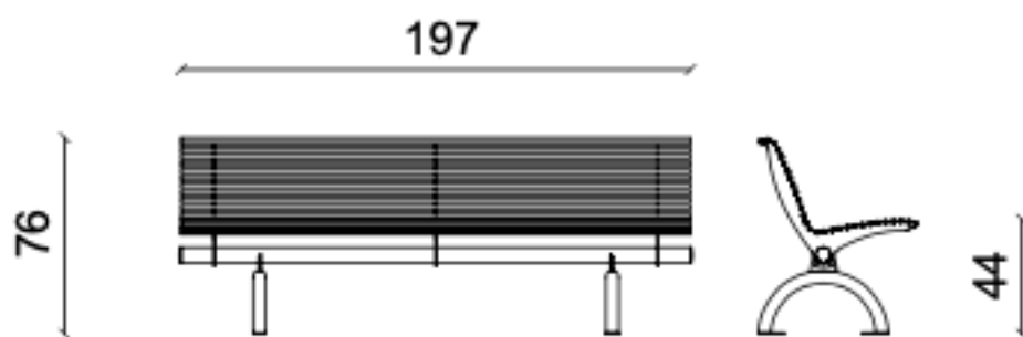
Bänk med ryggstöd
