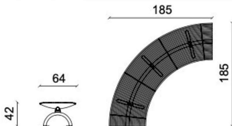
Svängd flat bänk
