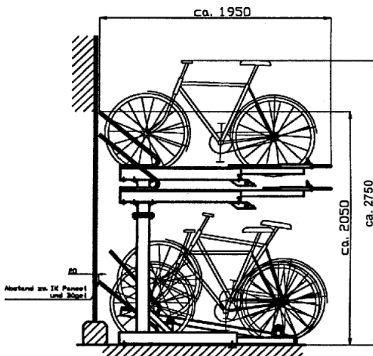
Doppelseitige Beschickung
