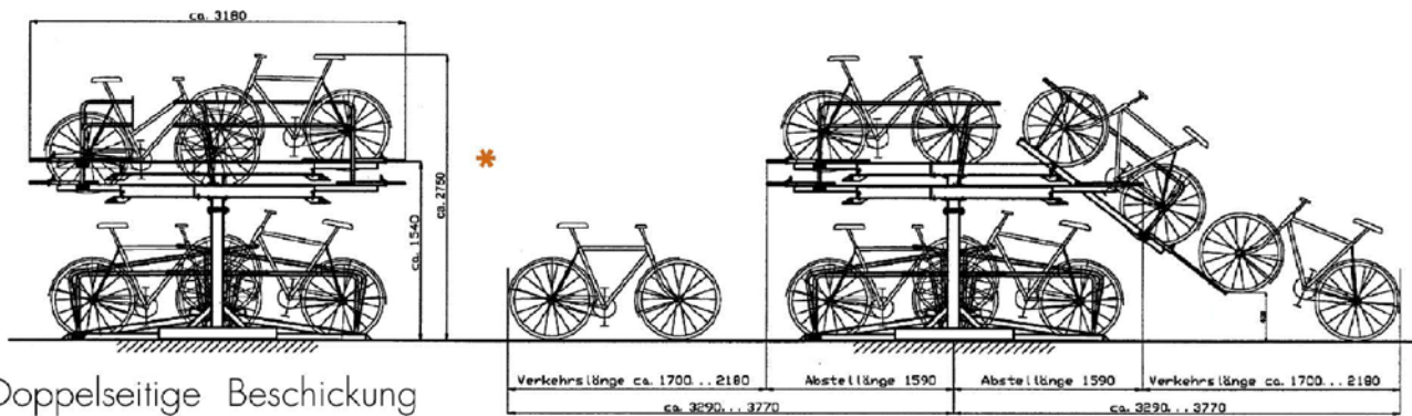
Einseitige Beschickung
