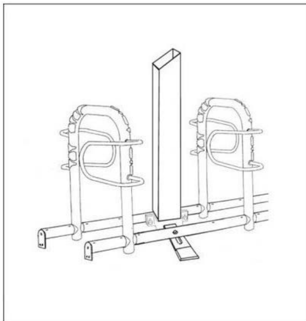
Fäst med stålfästen som förbinder cykelställets rörformade ram med stöden på en övertäckning.
